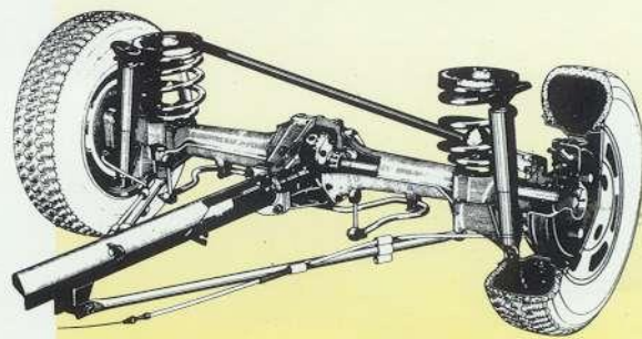
Diferencial autoblocante.
