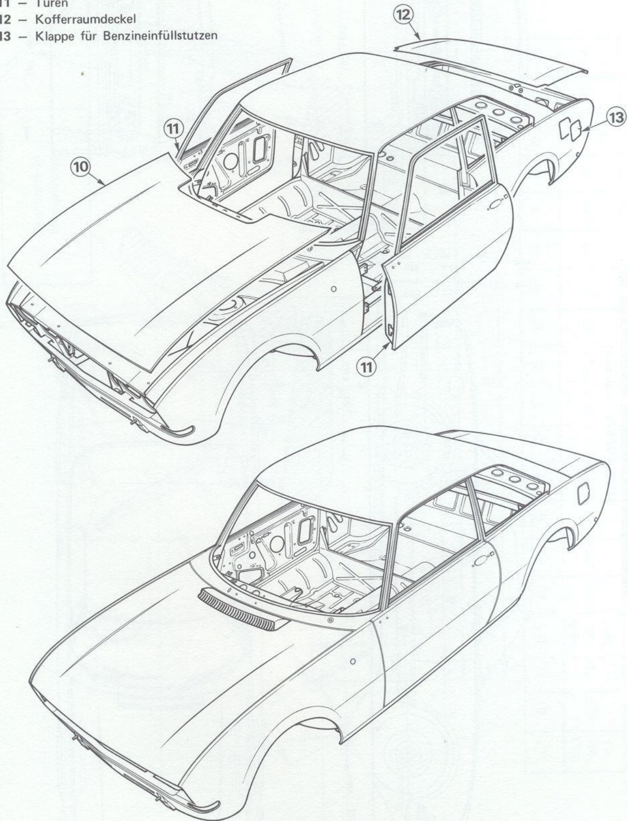
Karosserie des COUPES 504
