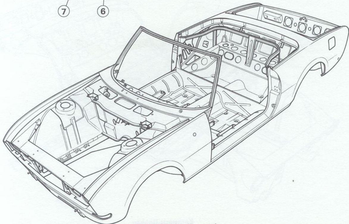
GANZSTAHL-Karosserie
