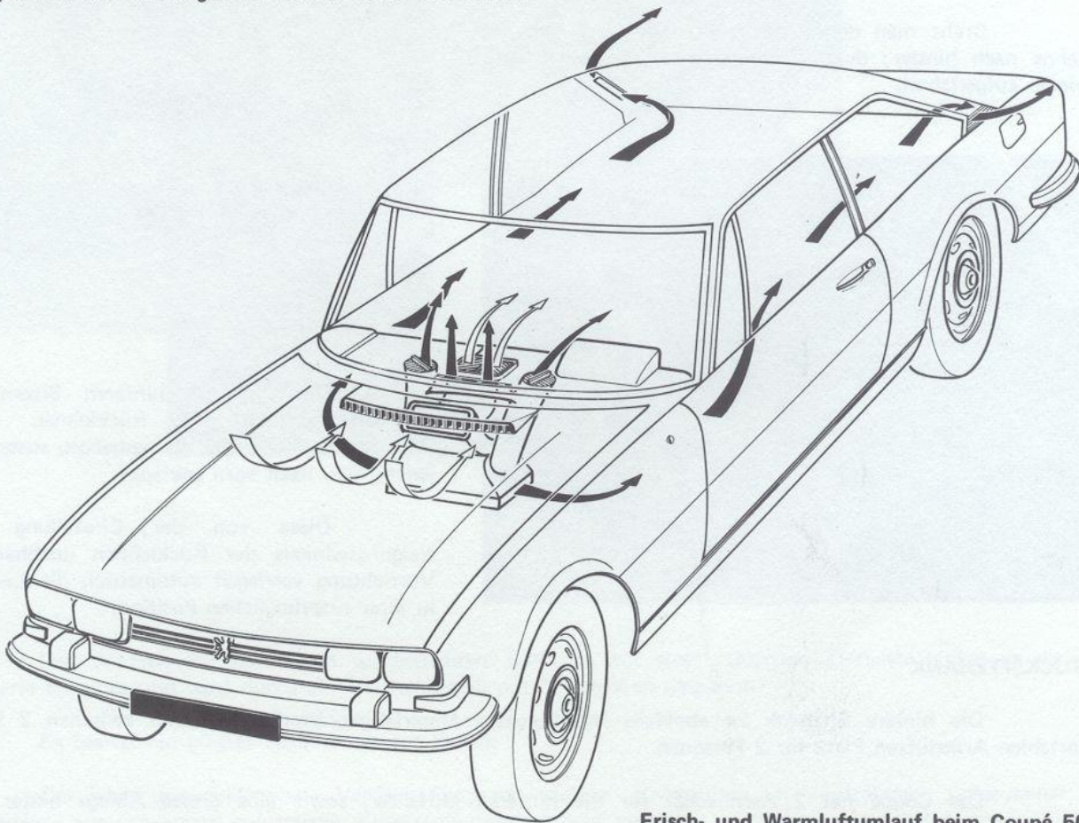
Frisch- und Warmluftumlauf beim Coupé 504
