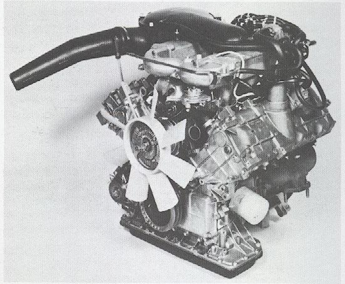
De nieuwe V6-injectie-motor heeft een cilinderinhoud van 2664 cc, geeft 144 DIN pk bij 5500 omw./min. en is goed voor een topsnelheid van 186 km.
